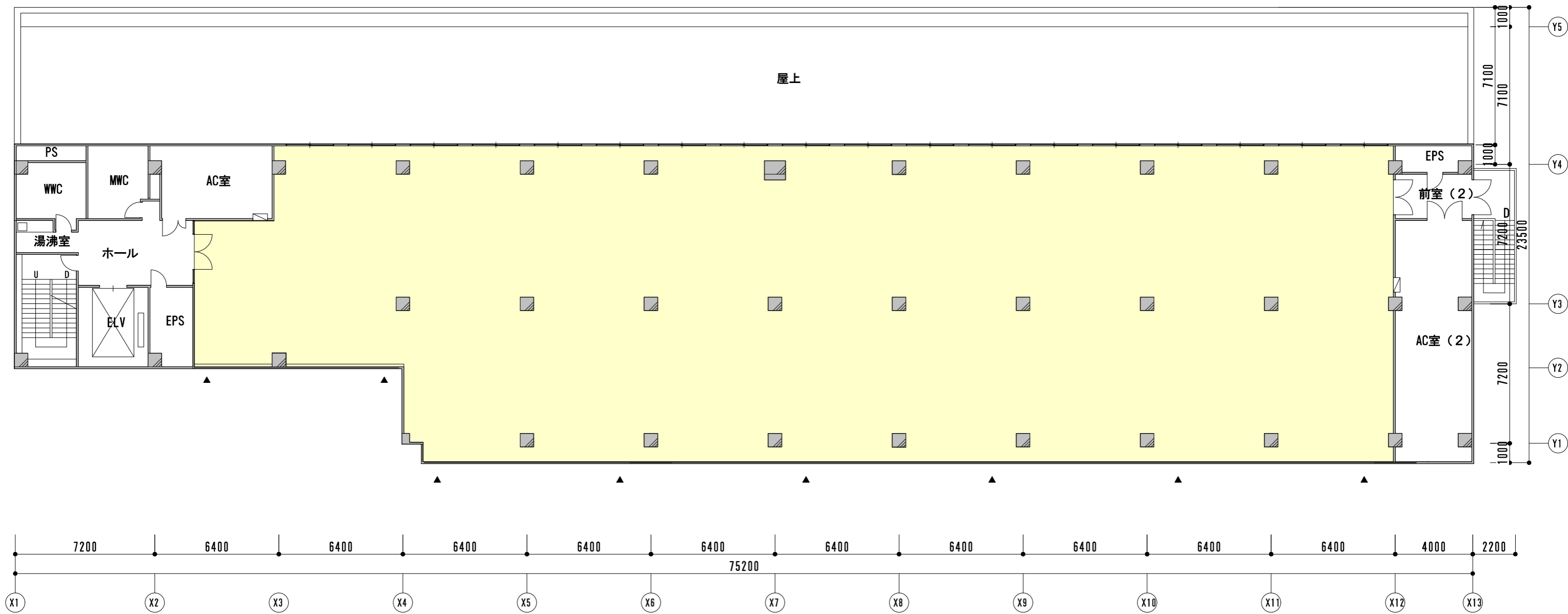
3階平面図 1 : 200
