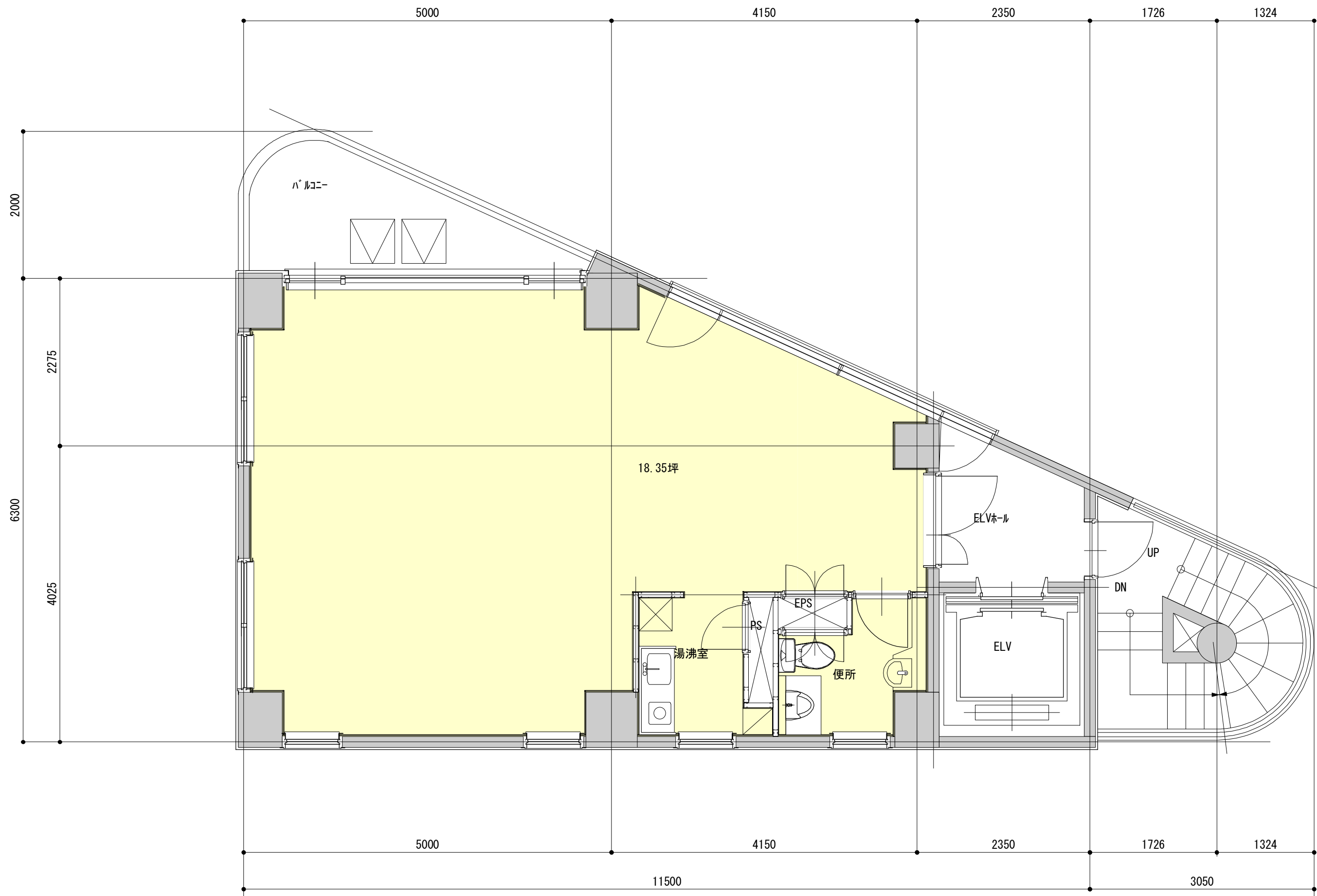
基準階平面図 1:50
