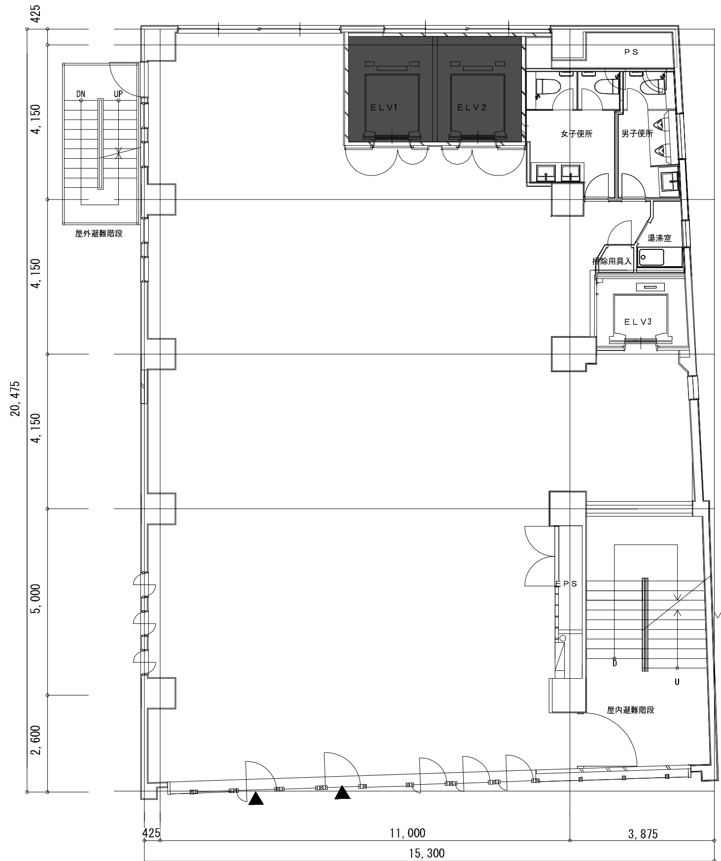
6階平面図 1:100
