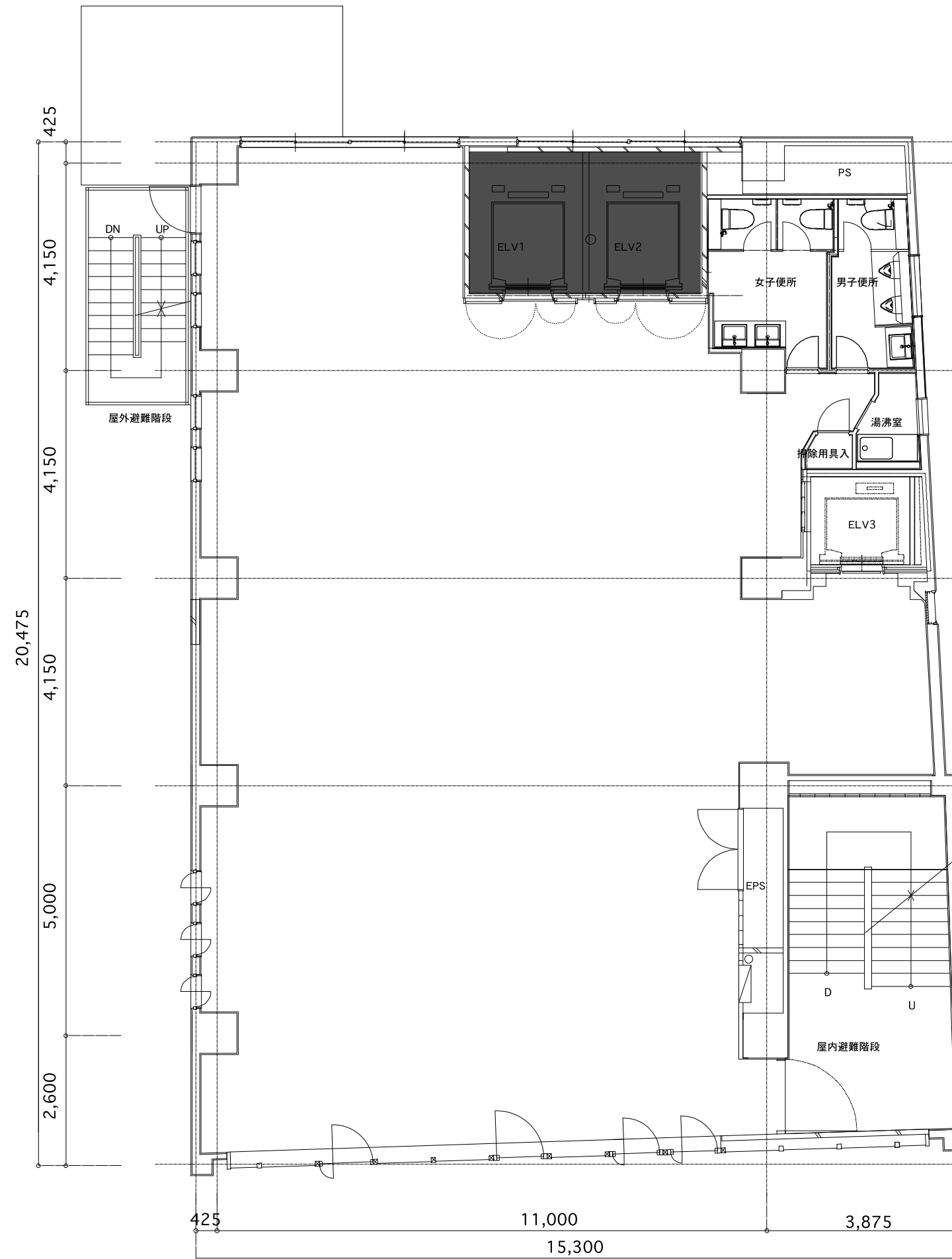
5階平面図 1:100
