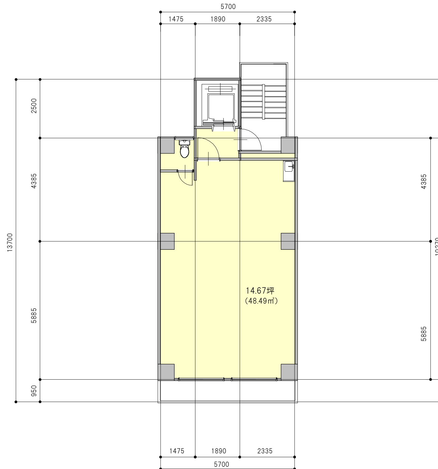
6階 平面図
