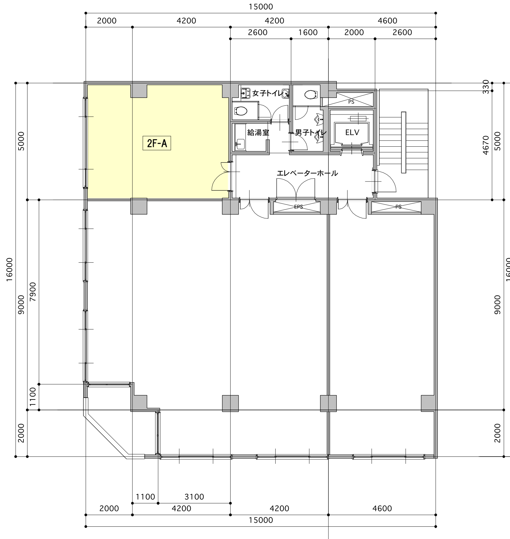
2階平面図 1:100
