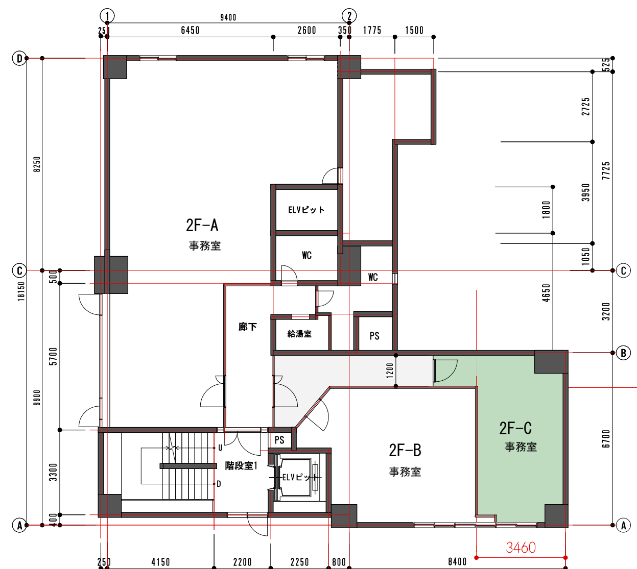
2階 平面図C
