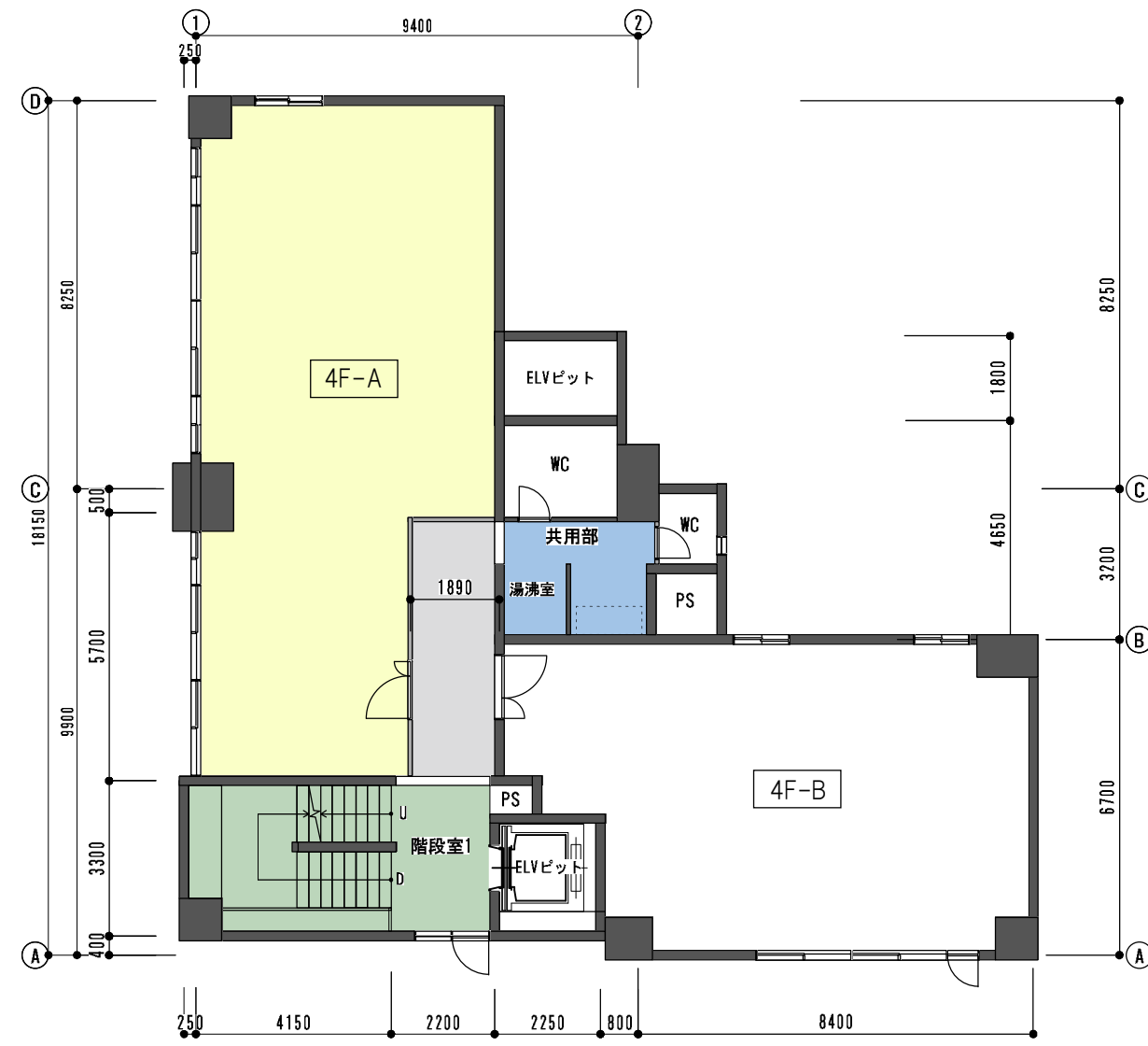
4階 平面図
