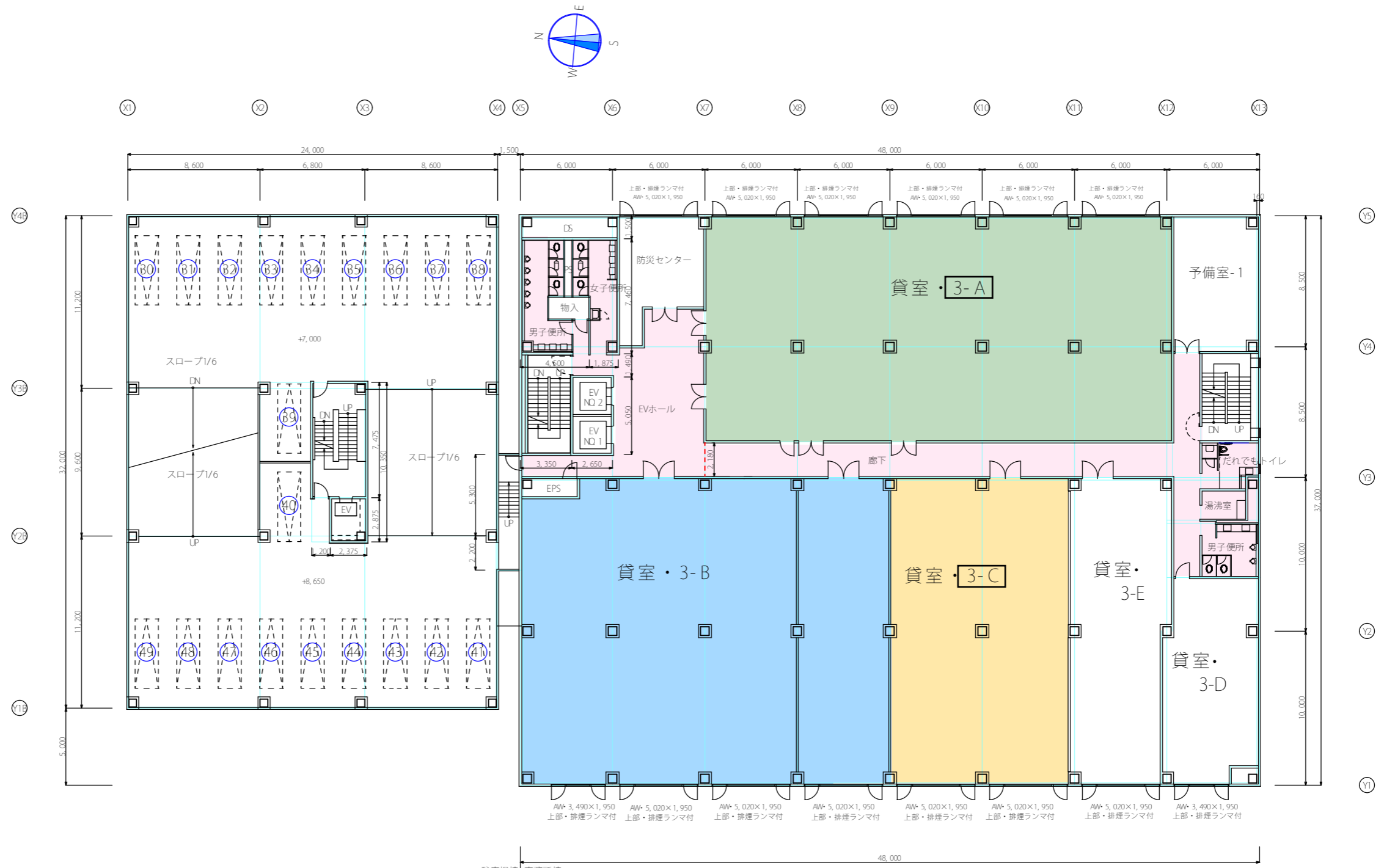
駐車場棟・3階平面図 3階駐車台数・20台
