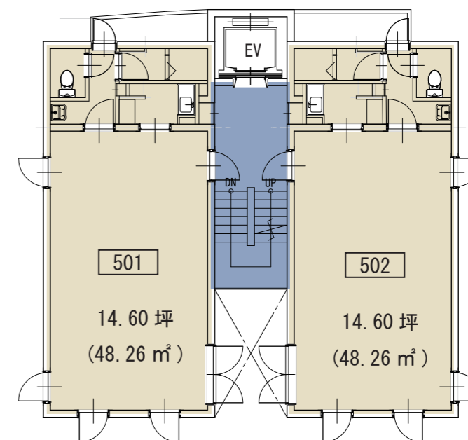
5階 平面図
