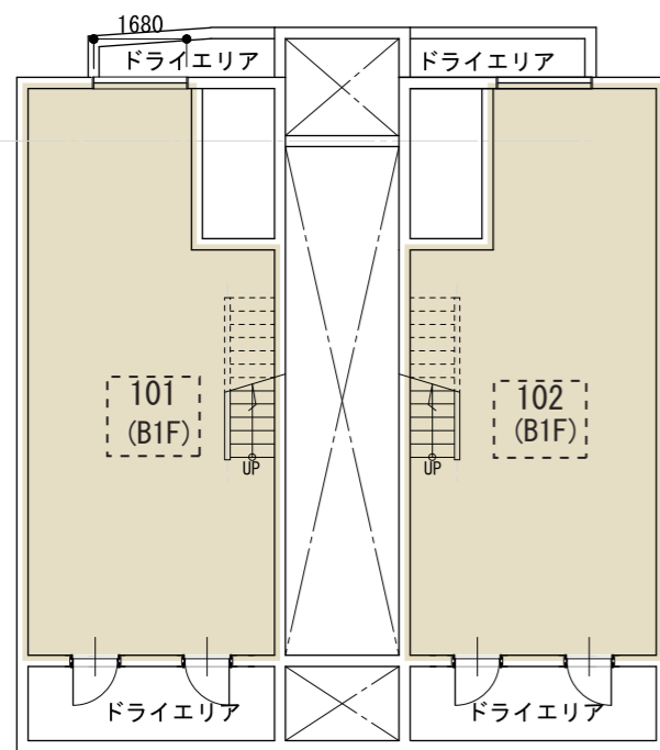
B1階平面図
