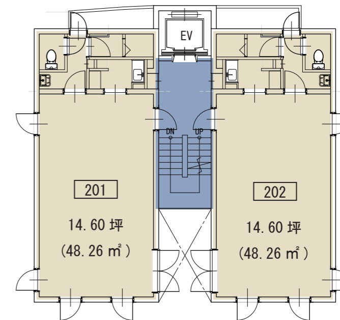
2階 平面図
