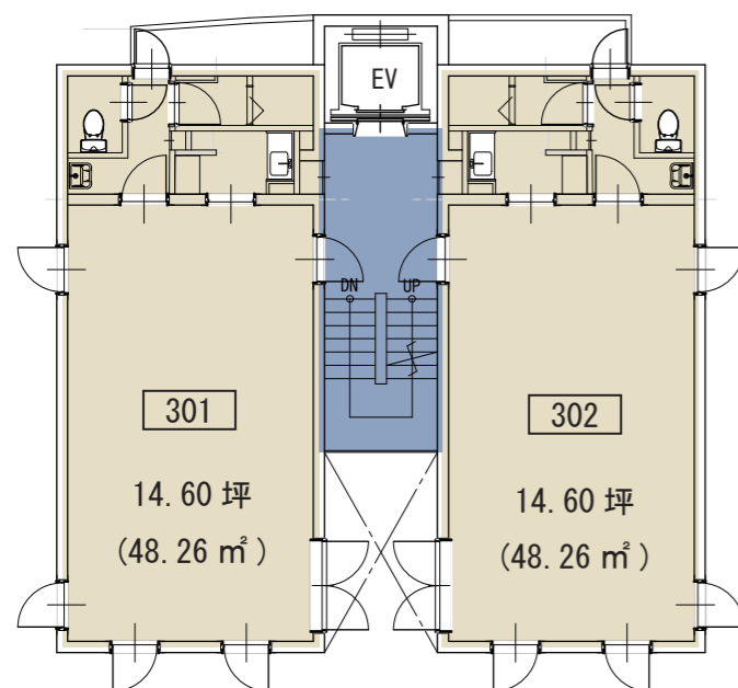
3階 平面図
