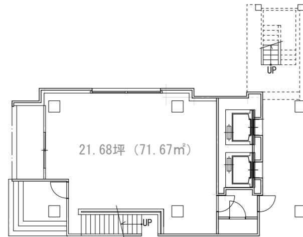
1階 平面図
