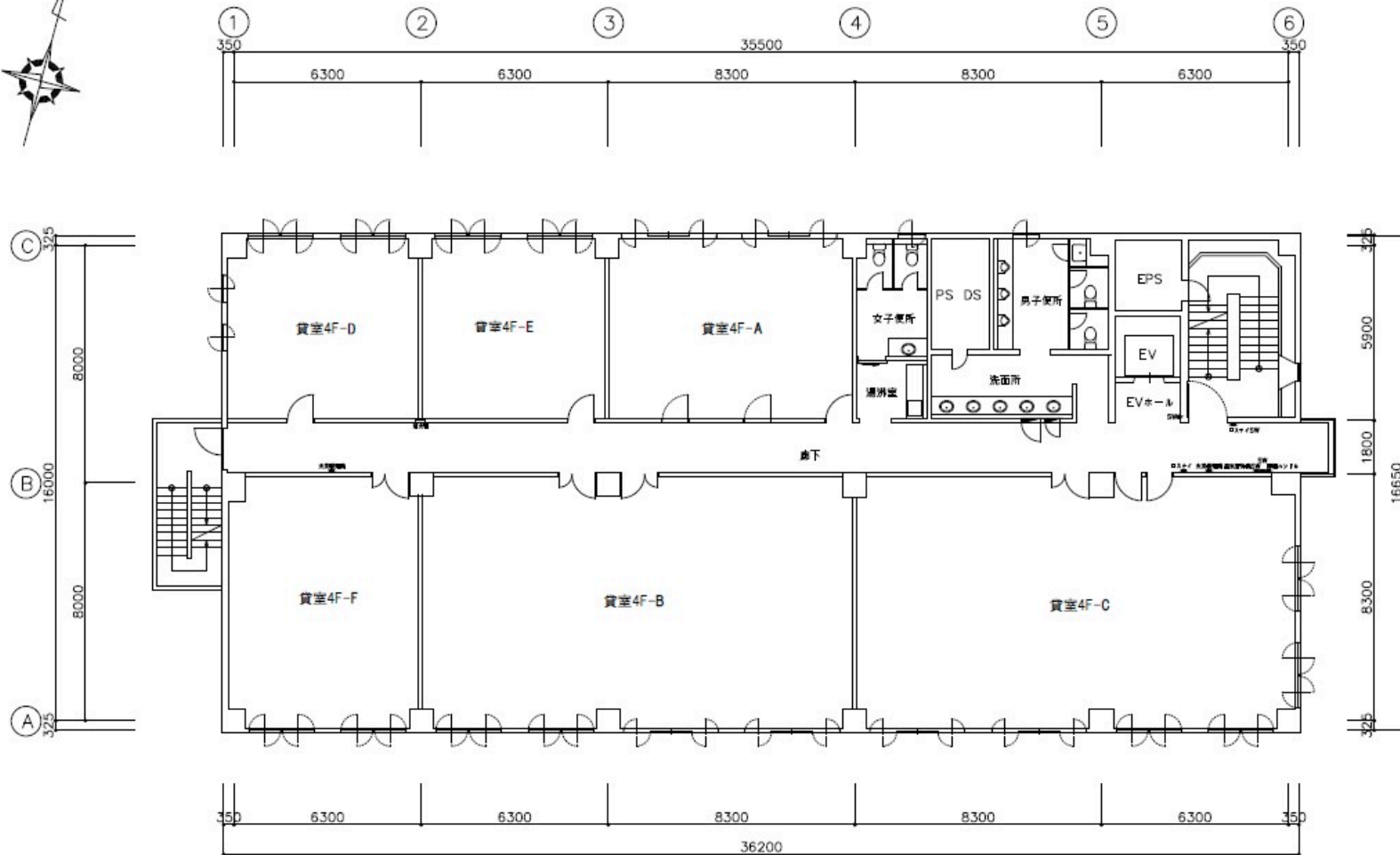
4階平面図
