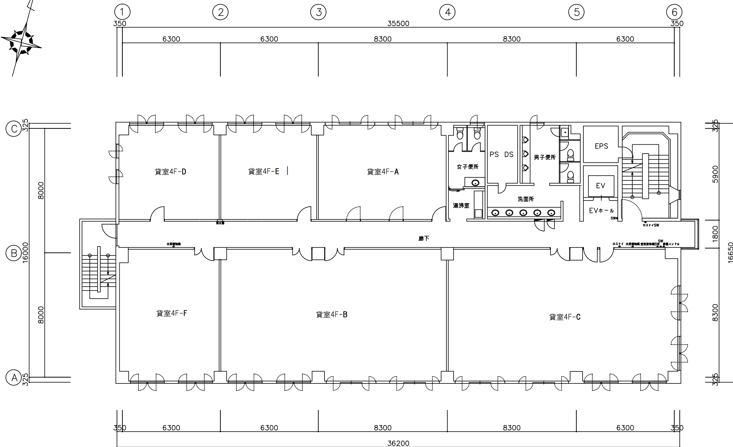
4階平面図
