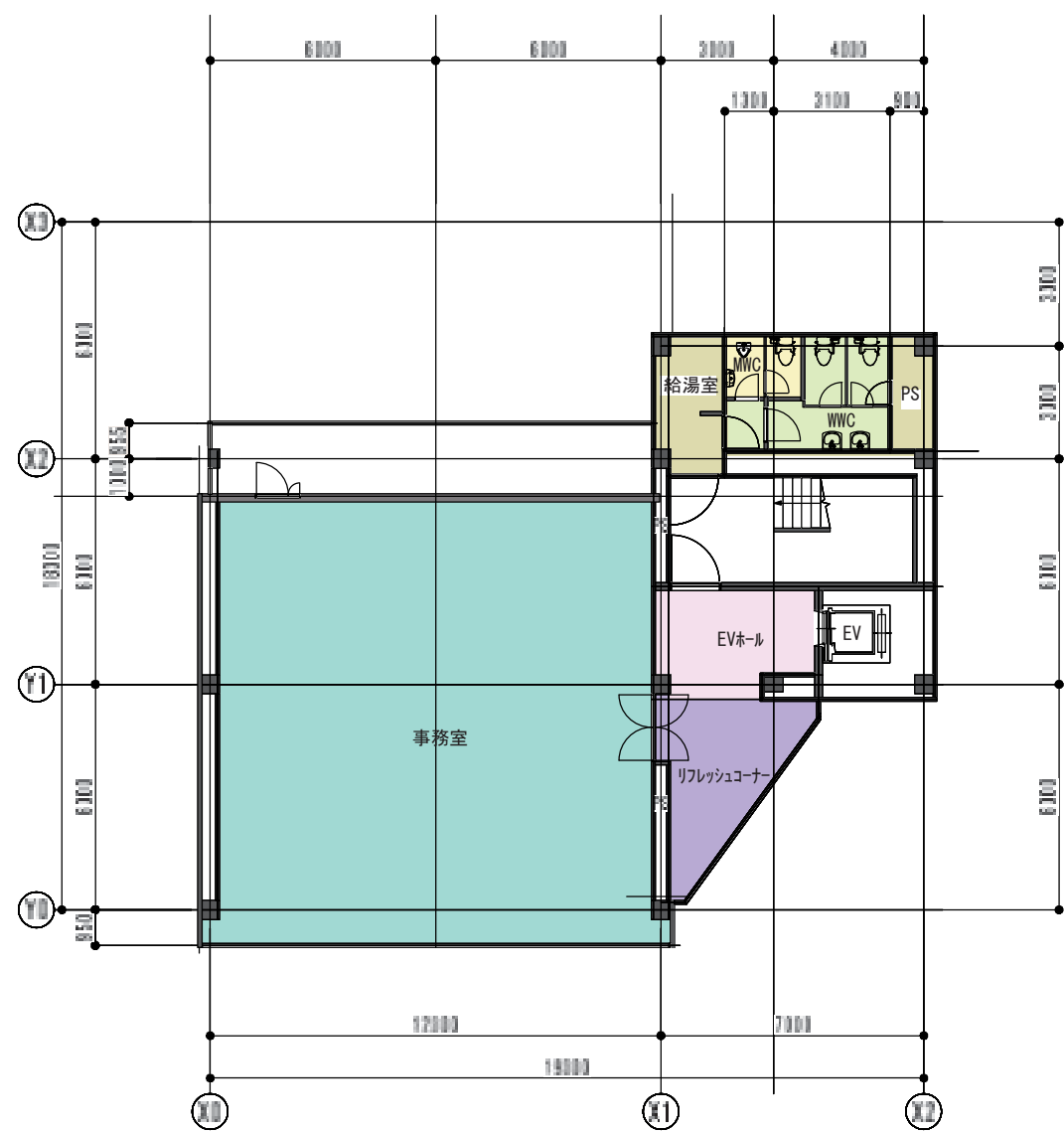
5階 平面図
